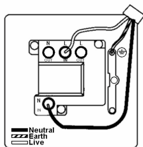
Wiring
